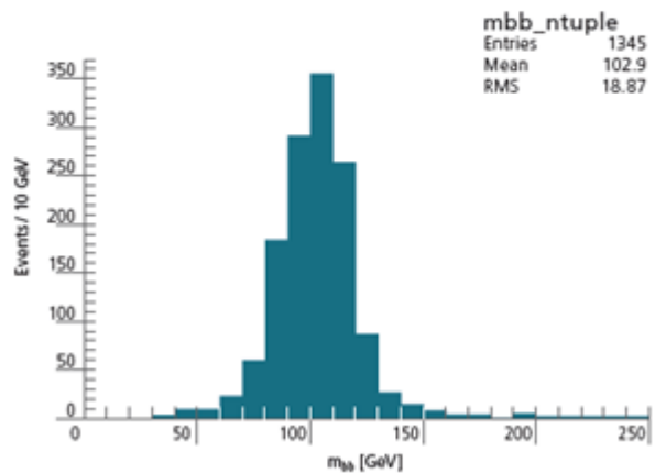
Invariant di-bjet mass
