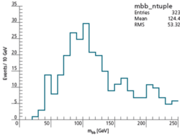
Invariant di-bjet mass
